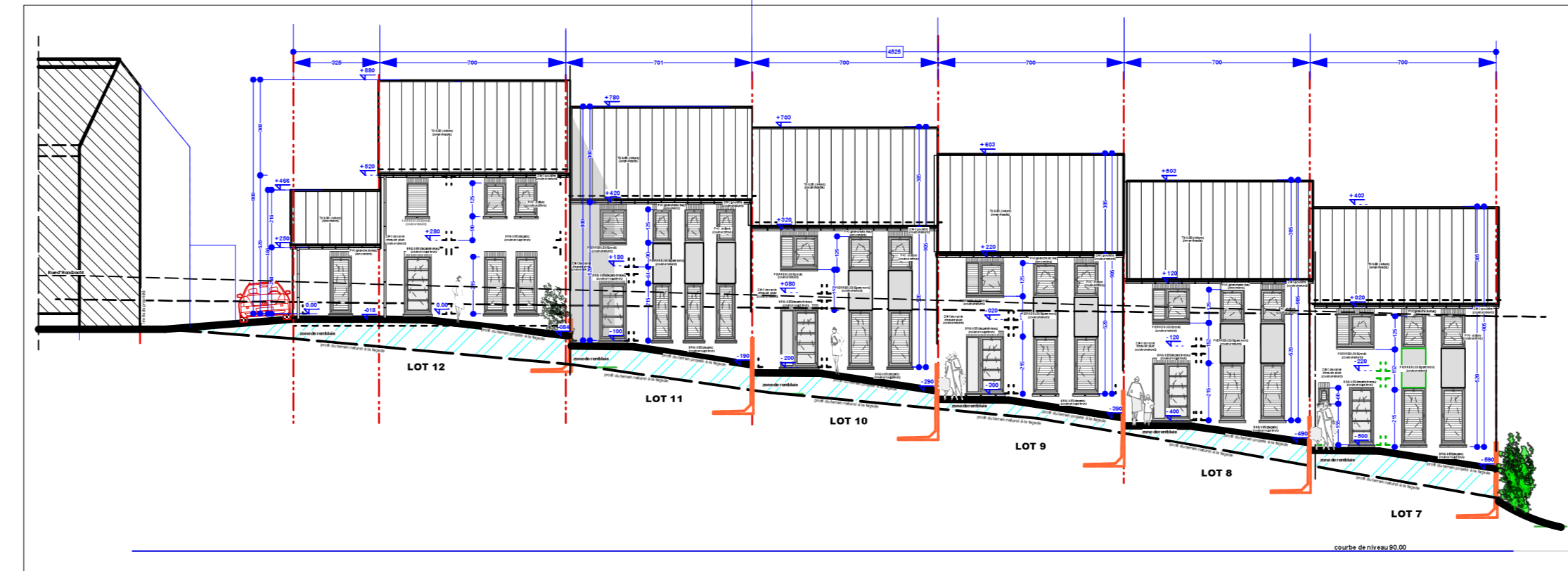
COUPE PROFIL 1 ECH 1/200
