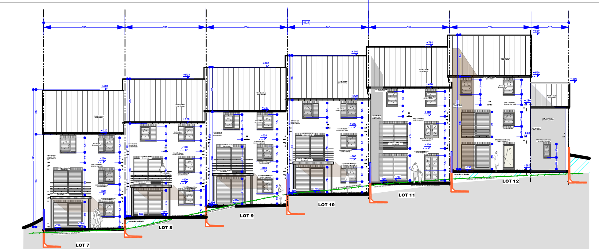
COUPE PROFIL 2 ECH 1/200
